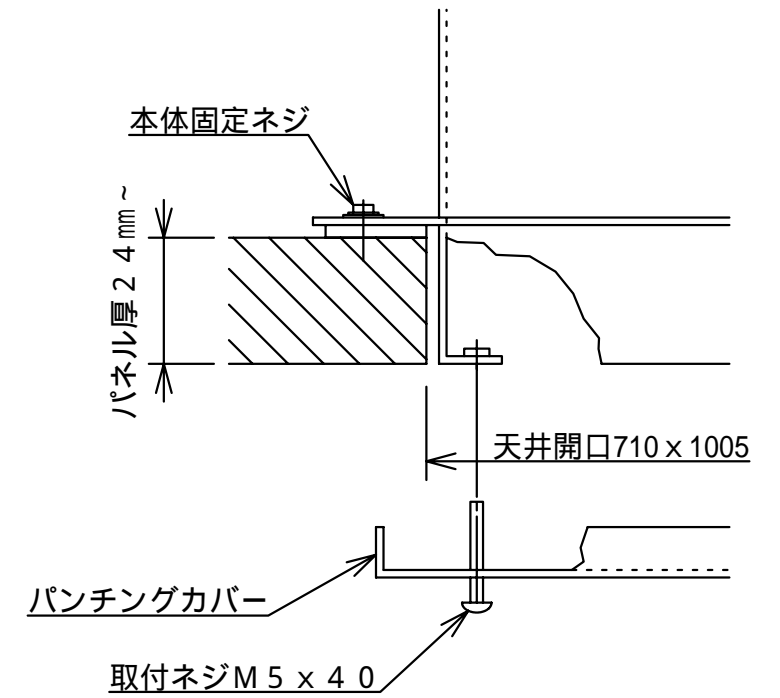
天井取付詳細図
